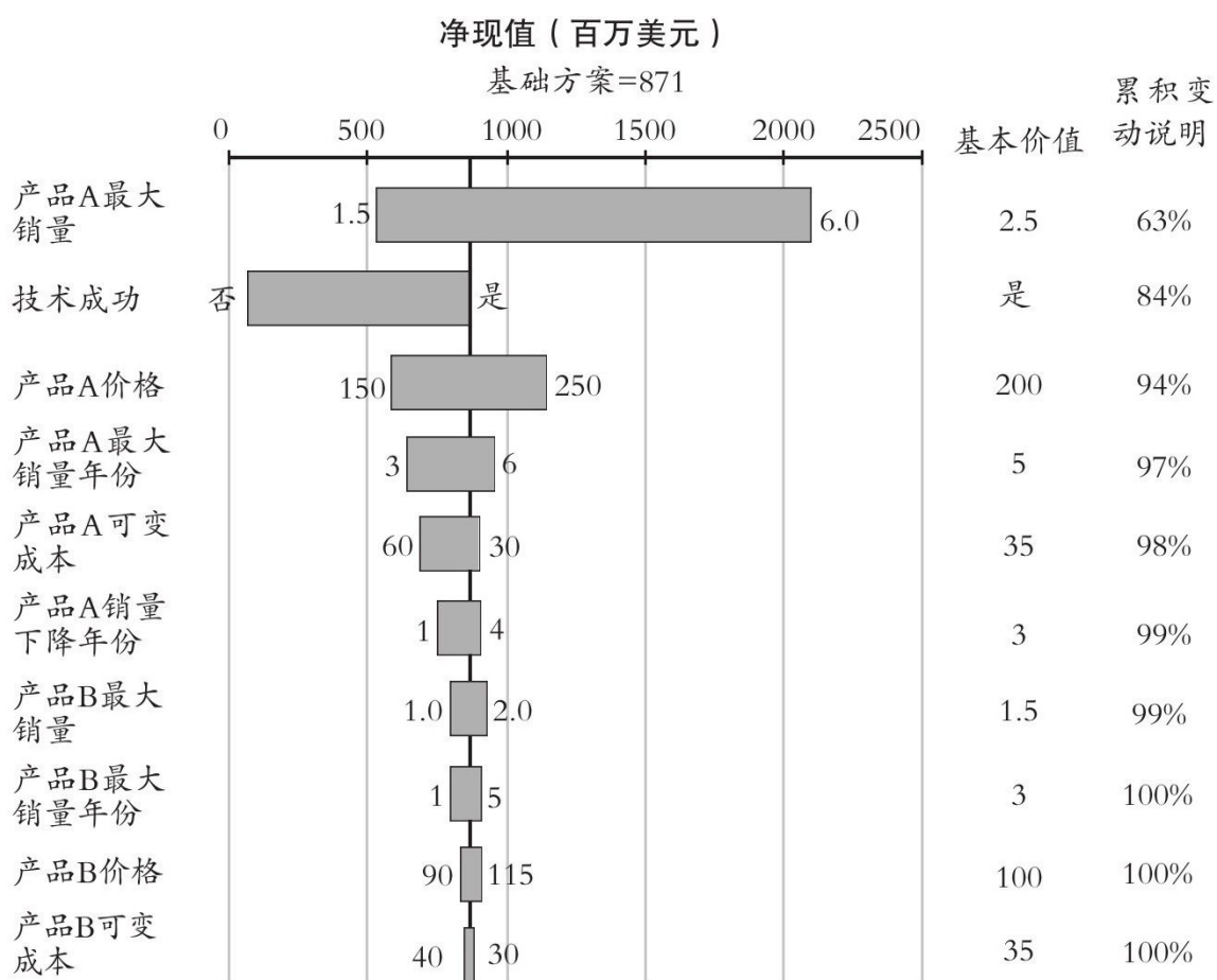
图8.5 典型商业选项的龙卷风图
