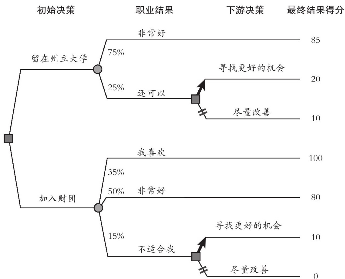
图13.5 加入罗宾的结果概率
